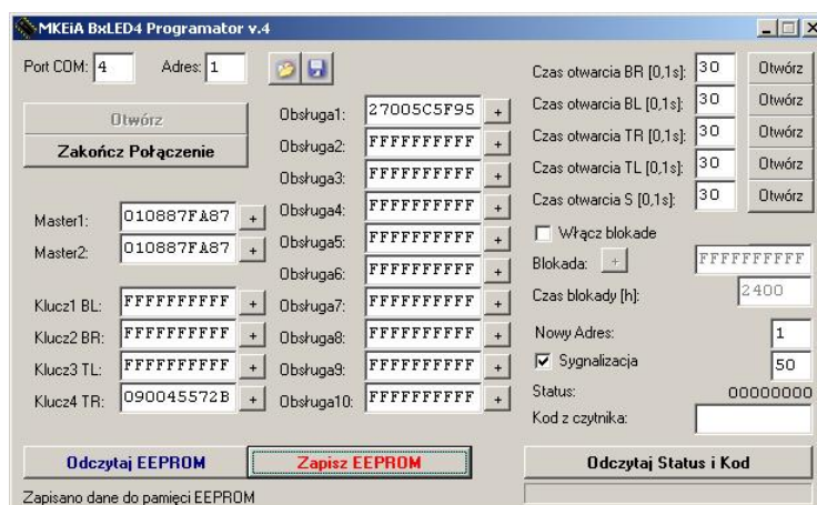
Rysunek nr 3 - Program BxLED4 Programator
